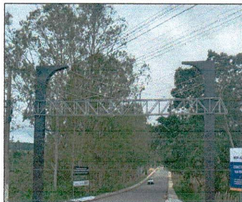
Foto 10: Estrutura metálica instalada.
